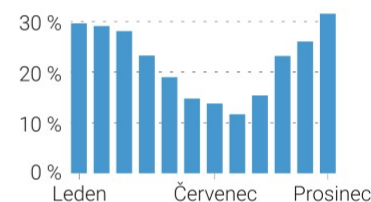
Průměrný koeficient využití větrných elektráren v letech 2015–2020
