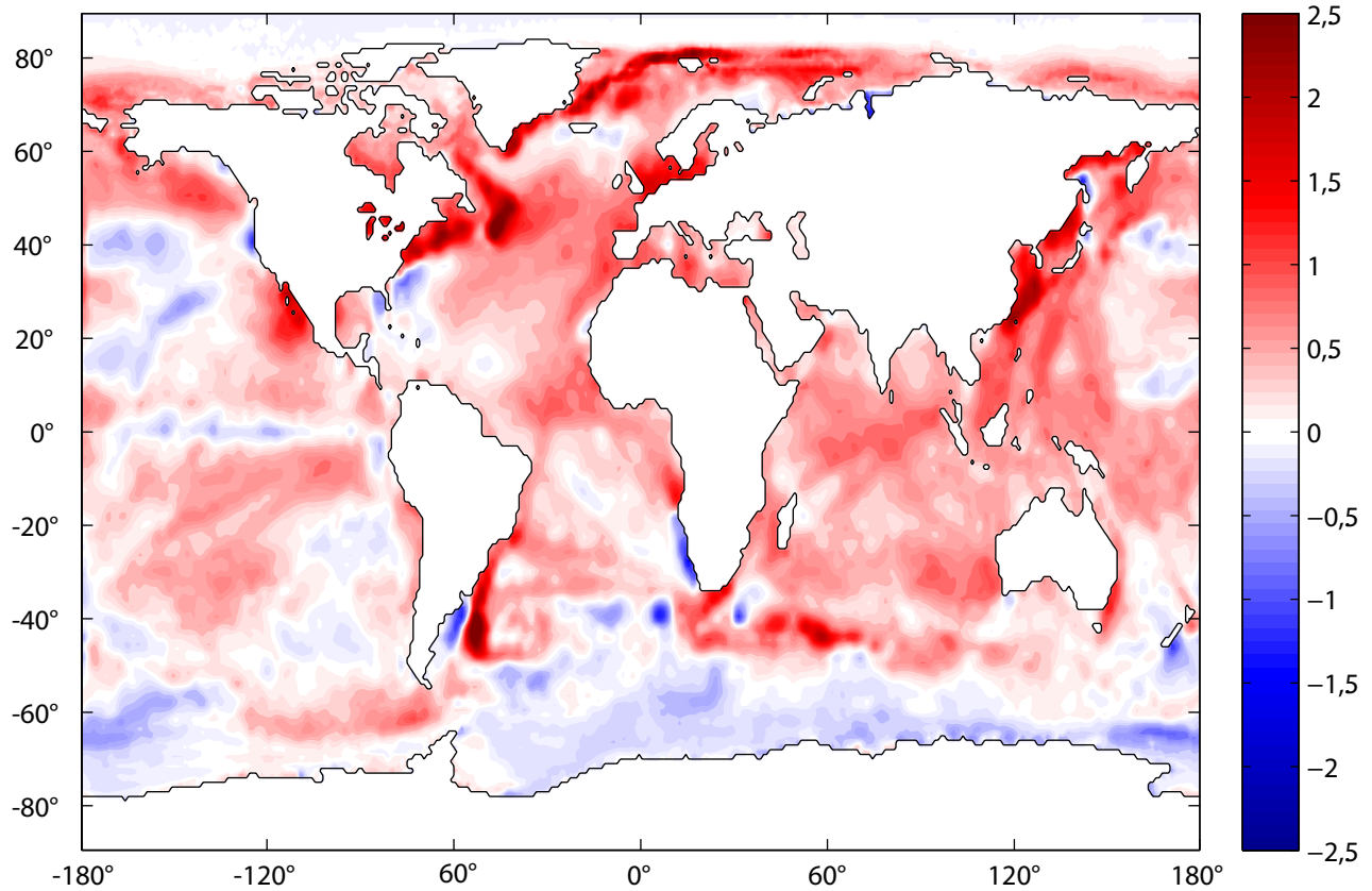
Trend v teplotě povrchů oceánů 1959 – 2008 / 1 K
