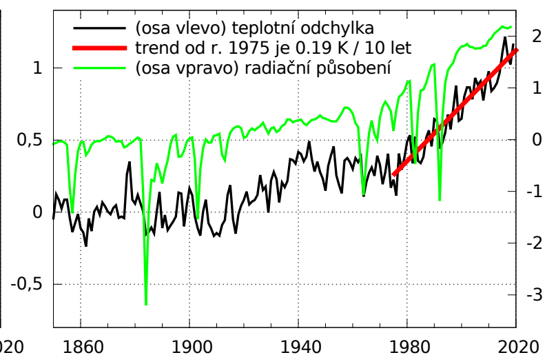
Glob. teplotní odchyly /K; rad. působení /( \text{W}/\text{m}^2 )
