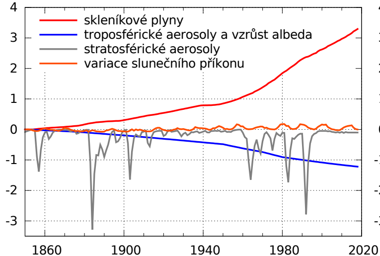
Jednotlivá radiační působení / ( \text{W}/\text{m}^2 )
