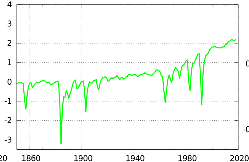
Celkové radiační působení / ( \text{W}/\text{m}^2 )
