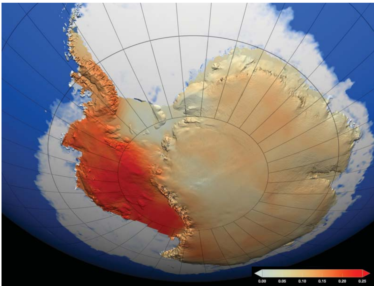
Obrázek 14. Trend průměrné roční teploty vzduchu ve °C/desetiletí v období let 1957–2006 ze Steig et al. 2009.
