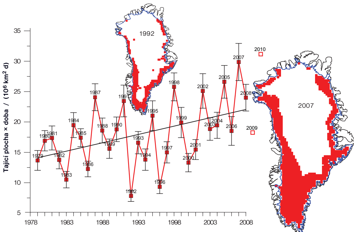
Obrázek 9. Podle pasivních mikrovlnných dat ze satelitů se celková plocha tání grónského ledového štítu v období let 1979 až 2008 zvětšila o 30 %, nejextrémnější tání bylo v roce 2007. Obecně je 33–55 % celkové ztráty hmoty z ledového štítu Grónska způsobeno táním na povrchu a odtokem. V roce 2007 docházelo k tání na zhruba 50 % celkové plochy ledového štítu. Malé tání v roce 1992 bylo způsobeno sopečnými aerosoly z Mt. Pinatubo, které byly příčinou krátkodobého globálního ochlazení (aktualizováno ze Steffen et al. 2008; pro 2009 a 2010 jsou uvedeny hrubé odhady dle Mote 2010, soukr. sdělení).
