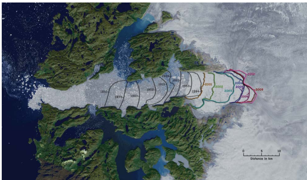
Obrázek 11. Plovoucí ledový jazyk představující výběžek Jakobshavn Isbrae směrem se již rozpadl. Jsou vyznačeny změny polohy čáry tání od roku 1851 do roku 2010, podkladový snímek v nepravých barvách je z 29. června 2009. Zdroj: http://svs.gsfc.nasa.gov/goto?3806 .
