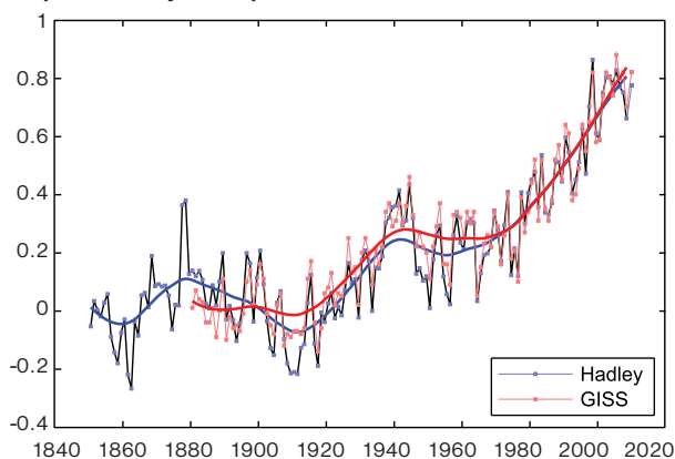
Teplota (odchylka od průměru 1880–1920) / 1 K
