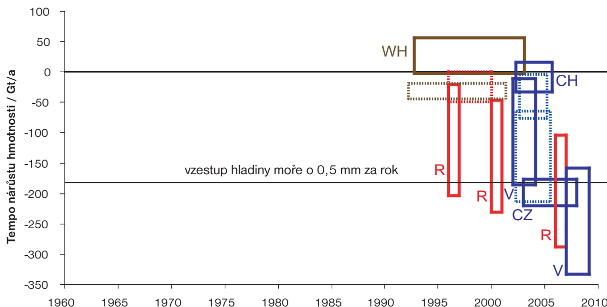
Obrázek 10. Odhady celkové bilance hmoty ledového štítu Antarktidy od roku 1992. Tečkované obdélníky představují odhady použité v IPCC AR4 (IPCC 2007). Obdélníky s plným obrysem jsou novější odhady (CH = Chen et al. 2006; WH = Wingham et al. 2006; R = Rignot et al. 2008b; CZ = Cazenave et al. 2009; V = Velicogna 2009).
