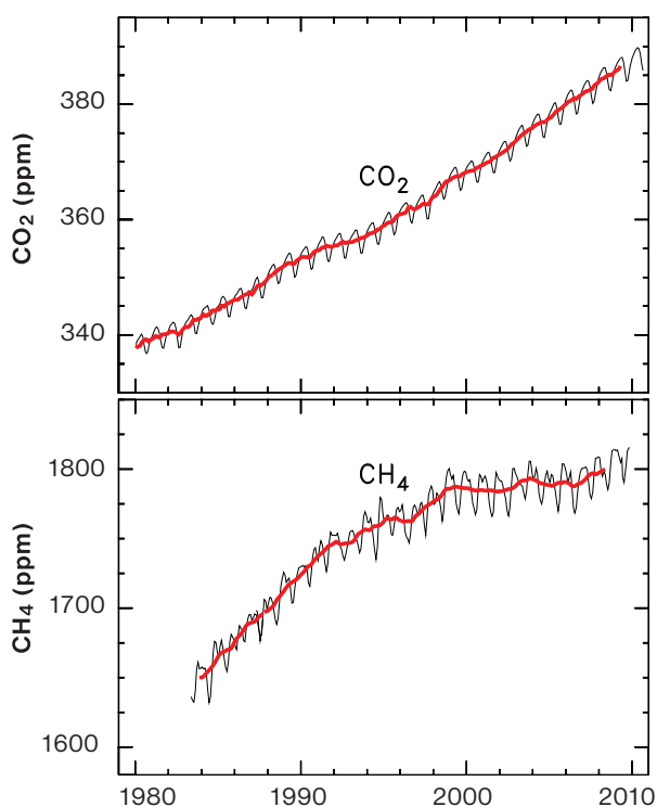
Obrázek 2. Koncentrace \text{CO}_2 (nahore) a \text{CH}_4 (dole) v atmosféře. Trendy po odstranění sezónního cyklu jsou vyznačeny červeně. \text{CO}_2 a \text{CH}_4 jsou dva nejdůležitější antropogenní skleníkové plyny. Data pocházejí z Earth System Laboratory amerického Národního úřadu pro oceán a atmosféru (NOAA). \text{CO}_2 je globální průměr. \text{CH}_4 je dle měření na stanici Mauna Loa.
