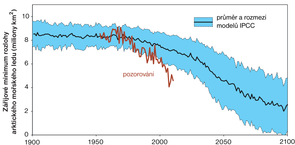
Obrázek 13. Pozorovaný (červená čára) a modelovaný rozsah mořského ledu v září v Arktidě v milionech čtverečních kilometrů. Plná černá čára udává střed souboru 13 modelů IPCC AR4, zatímco přerušované černé čáry představují jejich rozpětí. Podle Stroeve et al. (2007) aktualizováno zahrnutím dat do roku 2010.
