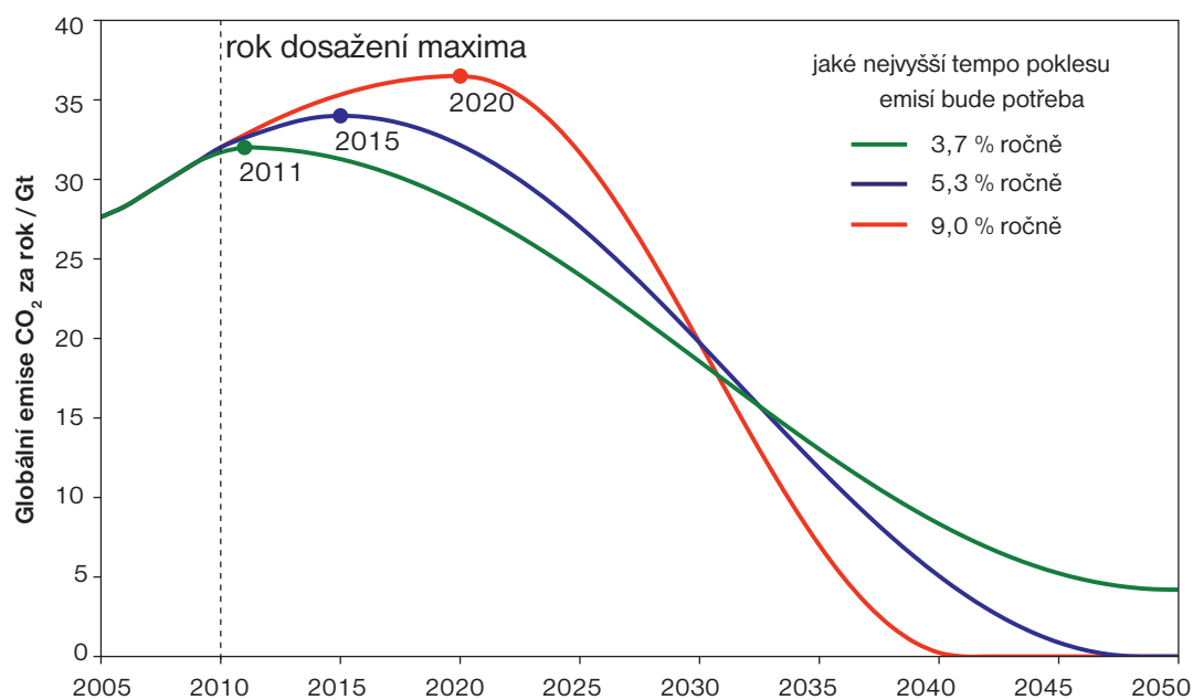
Obrázek 22. Příklady globálních emisních trajektorií takových, aby se úhrnné emise \text{CO}_2 za časové období 2010–2050 rovnaly 750 Gt (1 Gt C = 3,67 Gt \text{CO}_2 ). S touto hodnotou dosahuje pravděpodobnost omezení globálního oteplování na maximálně 2 °C hodnoty 67 %. Graf ukazuje, že čím později dosáhneme vrcholu emisí, tím strmější musí být jejich následné klesání. Na obrázku jsou varianty scénáře globálních emisí s různými roky vyvrcholení: 2011 (zeleně), 2015 (modře) a 2020 (červeně). K dosažení souladu s těmito křivkami bude zapotřebí maximální roční rychlosti poklesu (vzhledem k roku 2008) 3,7 % (zelená), 5,3 % (modrá) nebo 9,0 % (červená). (Zdroj: Vědecký poradní orgán německé spolkové vlády „Globální změna životního prostředí“; WBGU 2009.)
