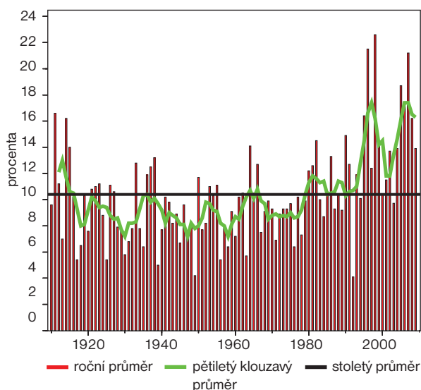
Index klimatických extrémů: USA, srážky celoroční 1910–2009
