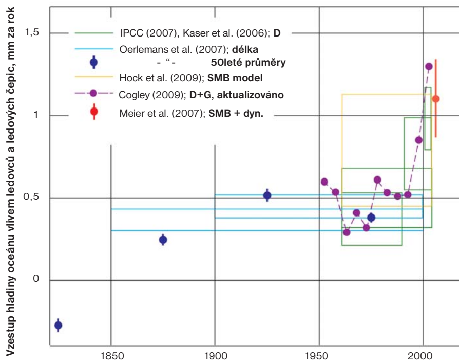
Obrázek 7. Odhady toho, kolik přispívají ledovce a ledové čepice ke globální změně výšky mořské hladiny, v milimetrech za rok. (Metody: D znamená přímá měření sněhové pokrývky ledu, G geodetické dálkové zjišťování objemu ledu, SMB je modelování bilance hmotnosti povrchové vrstvy, dyn. zahrnuje i změny v dynamice odtoku ledu.)
