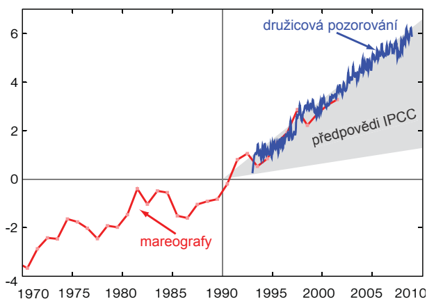
Obrázek 16. Změna výšky hladiny v období 1970–2010. Údaje z mareografů jsou vyznačeny červeně (Church a White 2006) a satelitní data moře (Cazenave et al. 2008). Pro srovnání jsou šedým stínováním zobrazeny projekce Třetí hodnotící zprávy IPCC.
