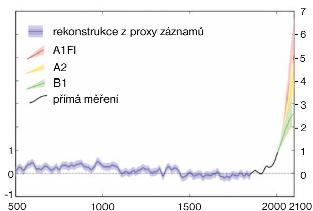
Globální teplota vzhledem k období 1800–1900 (°C)
