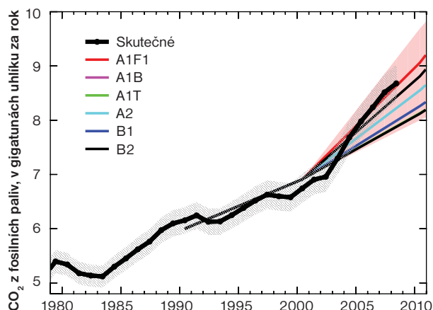
Obrázek 1. Pozorované celosvětové emise CO 2 ze spalování fosilních paliv a výroby cementu ve srovnání s emisními scénáři IPCC (Le Quéré et al. 2009). Pozorování až do roku 2006 pocházejí z Centra pro rozbor informací o oxidu uhličitém (CDIAC) při Ministerstvu energetiky USA. V letech 2007 a 2008 vycházejí z ekonomických údajů BP. Emisní scénáře jsou zprůměrovány přes rodiny scénářů představené v Nakicenovic et al. (2000). Stínovaná plocha pokrývá všechny scénáře používané IPCC k projekcím změny klimatu. Emise v roce 2009 nepřekročily hodnotu platnou pro rok 2008.
