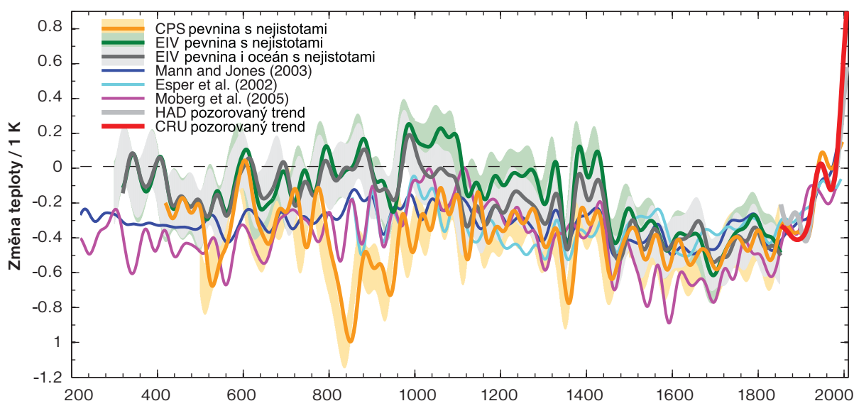
Obrázek 19. Porovnání různých rekonstrukcí teploty na severní polokouli zobrazených s odhadovanými 95% intervaly spolehlivosti (z Mann et al. 2008).
