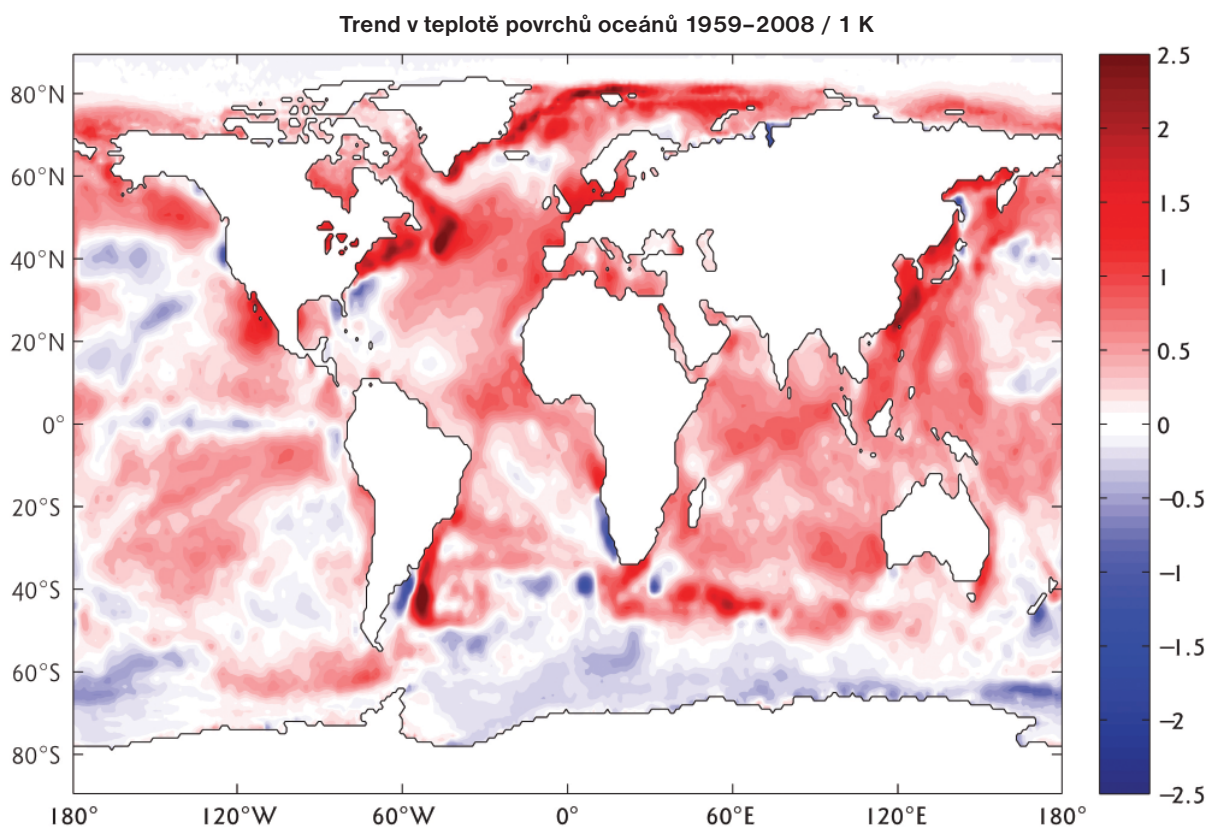
Obrázek 15. Dlouhodobá změna teploty povrchu moře (SST) za padesátileté období let 1959–2008 vypočtená fitováním lineárního trendu do 50 let měsíčních dat o SST v každém bodu sítě. Pole SST pocházejí ze souboru dat Hadleyho centra popsaného v Rayner et al. (2006).
