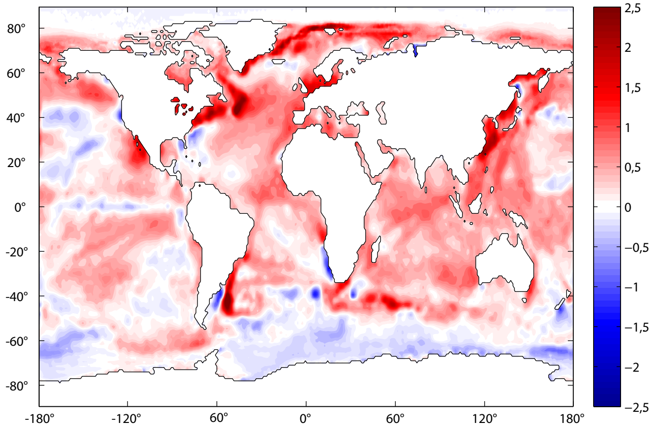
Trend v teplotě povrchů oceánů 1959 – 2008 / 1 K
