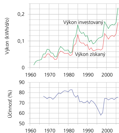
Obrázok 26.17 Účinnosť štyroch uskladňovacích zariadení vo Veľkej Británii.
