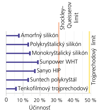
Obrázok 6.18 Účinnosť dnes dostupných solárnych fotovoltaických modulov. V texte predpokladám, že strešná fotovoltaika má účinnosť 20%, a že pozemné inštalácie fotovoltaiky majú 10% účinnosť. V mieste, kde je priemerný tok prichádzajúceho žiarenia 100 W/m^2 , panely s účinnosťou 20% vyrobia 20 W/m^2 .
