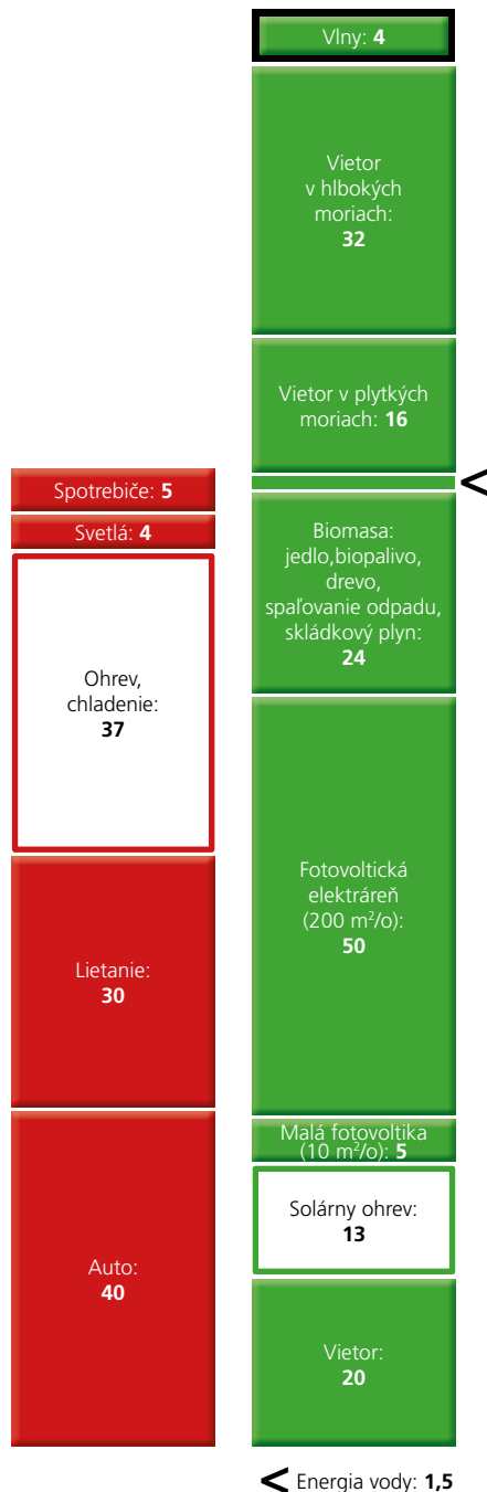
Obrázok 12.1 Vlny.
