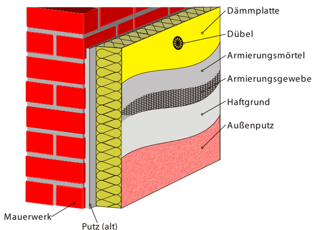
Schematisch dargestellt der Schichtaufbau eines Wärmedämmverbundsystems
