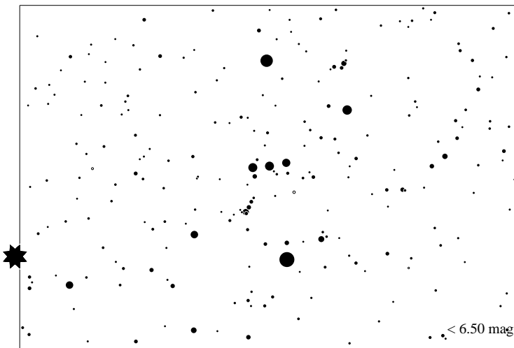
Mapky pro Globe at Night ( globe.hvezdarna.cz ) 22. 3., 20 h (začíná astron. noc), velmi průzračný vzduch. Orionův pás je 30^\circ nad JZ, nejjasnější stálice Sirius je těsně vlevo od vymezené oblasti. Pro světlejší nebe udáváme jen počty hvězd v ní viditelných: 11 pro limit 3 mag , 5 pro 2 mag , 2 pro 1 mag .
