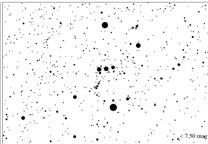
Mapky pro Globe at Night ( globe.hvezdarna.cz ) 22. 3., 20 h (začíná astron. noc), velmi průzračný vzduch. Orionův pás je 30^\circ nad JZ, nejjasnější stálice Sirius je těsně vlevo od vymezené oblasti. Pro světlejší nebe udáváme jen počty hvězd v ní viditelných: 11 pro limit 3 mag , 5 pro 2 mag , 2 pro 1 mag .
