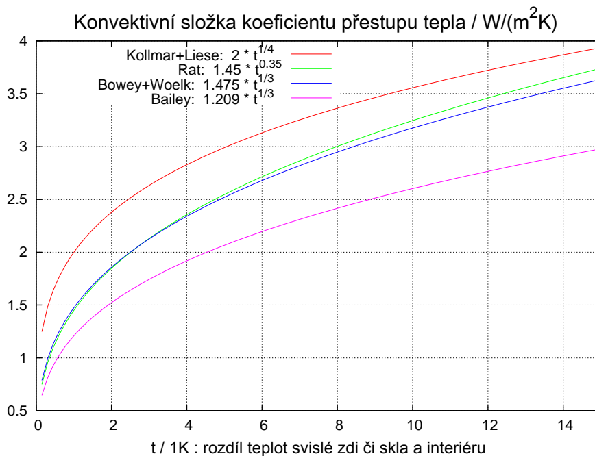
Obrázek 2.2: Konvekce na interiérové straně
