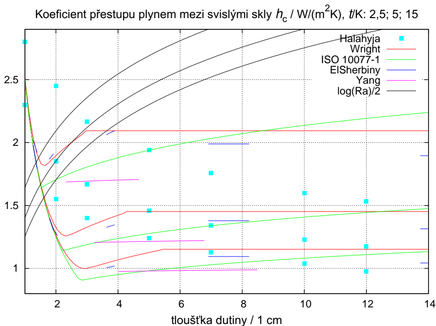
Obrázek 2.7: Neradiační složka přestupu tepla, i pro tlusté dutiny. Zdroje: Halahya [21, str. 64], Wright: [68], ISO 10077-1: [6], EISherbiny: [11], Yang: [70]. Nejstarší zdroj Halahya téměř jistě přeceňuje vliv konvekce u tenkých dutin, ISO 10077-1 a Wright naopak jej přeceňují naopak u tlouštěk nad 10 cm.
