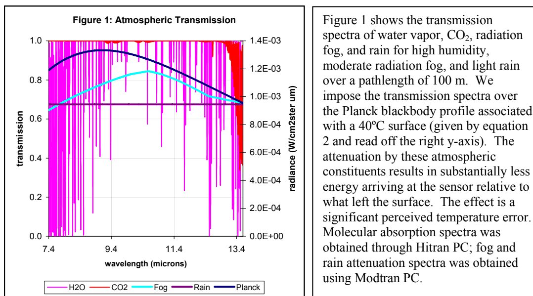
Obrázek 3.2: Transmittance ovzduší při pozorování skrze vrstvu tloušťky 100 m. Křivkami je znázorněn možný vliv mlhy a deště. Na pravé straně je škála spektrálních září pro černé těleso teploty 40 °C / ( 10^{-4} \text{ W}/(\text{m}^2 \text{ sr } \mu\text{m}) ) (převzato z [10]) (viz text str. 42)
