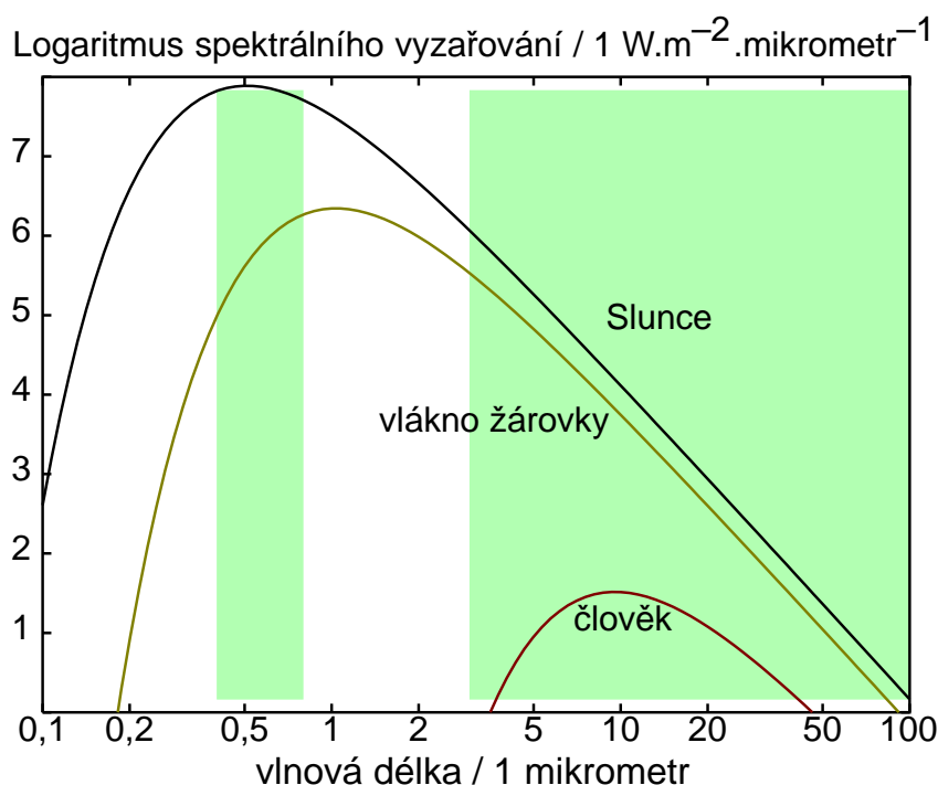
Obrázek 2.1: „Planckovy křivky“ v logaritmickém zobrazení. Stínováním jsou odleva vyznačeny postupně oblasti ultrafialová, viditelná, infračervená krátkovlnná a dlouhovlnná.
