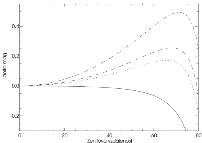
Obrázek 4: Teoretické průběhy závislosti jas nebe na zenitové vzdálenosti pro extinkční koeficient k = 0.35 a různé hodnoty parametru f (viz část 4.1) – 0.3 (plně), 0.6 (čárkovaně-krátké čárky), 0.7 (čárkovaně-dlouhé čárky) a 1.0 (čerchovaně)
