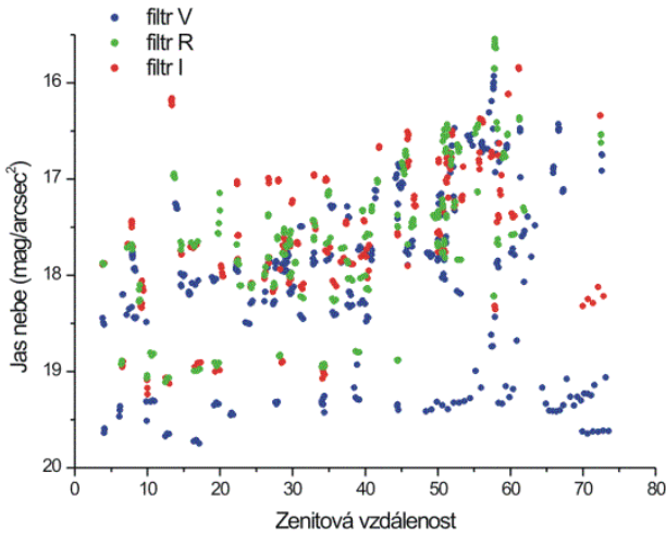
Obrázek 5: Naměřená závislost hvězdné velikosti čtvereční vteřiny nebe na zenitové vzdálenosti
