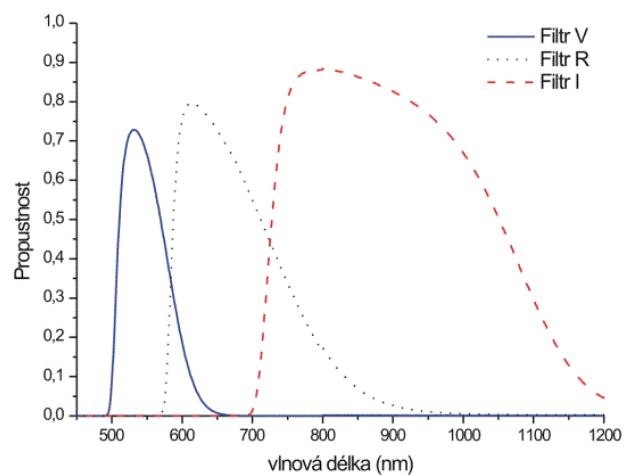
Obrázek 1: Křivky propustnosti filtrů použité CCD kamery
