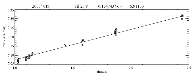
Obrázek 3: Příklad určení extinkčního koeficientu v noci 19./20. 7. 2003 ve filtru V
