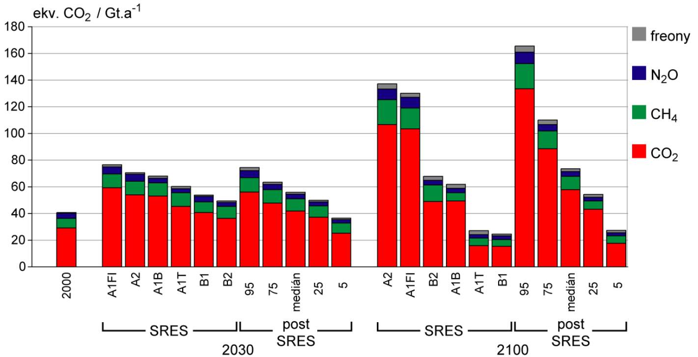
Obrázek SPM.4: Globální emise skleníkových plynů za rok 2000 a projektované referenční emise pro roky 2030 a 2100 dle scénářů SRES IPCC a dle odborné literatury publikované po vydání scénářů SRES (post-SRES). Obrázek ukazuje emise podle šesti ilustrativních scénářů SRES. Rovněž znázorňuje rozložení četnosti emisí scénářů publikovaných po SRES (percentily 5, 25, medián, 75, 95), jak uvádí kapitola 3. Freony zahrnují částečně a plně fluorované uhlovodíky a SF 6 [1.3, 3.2, Obrázek 1.7].
