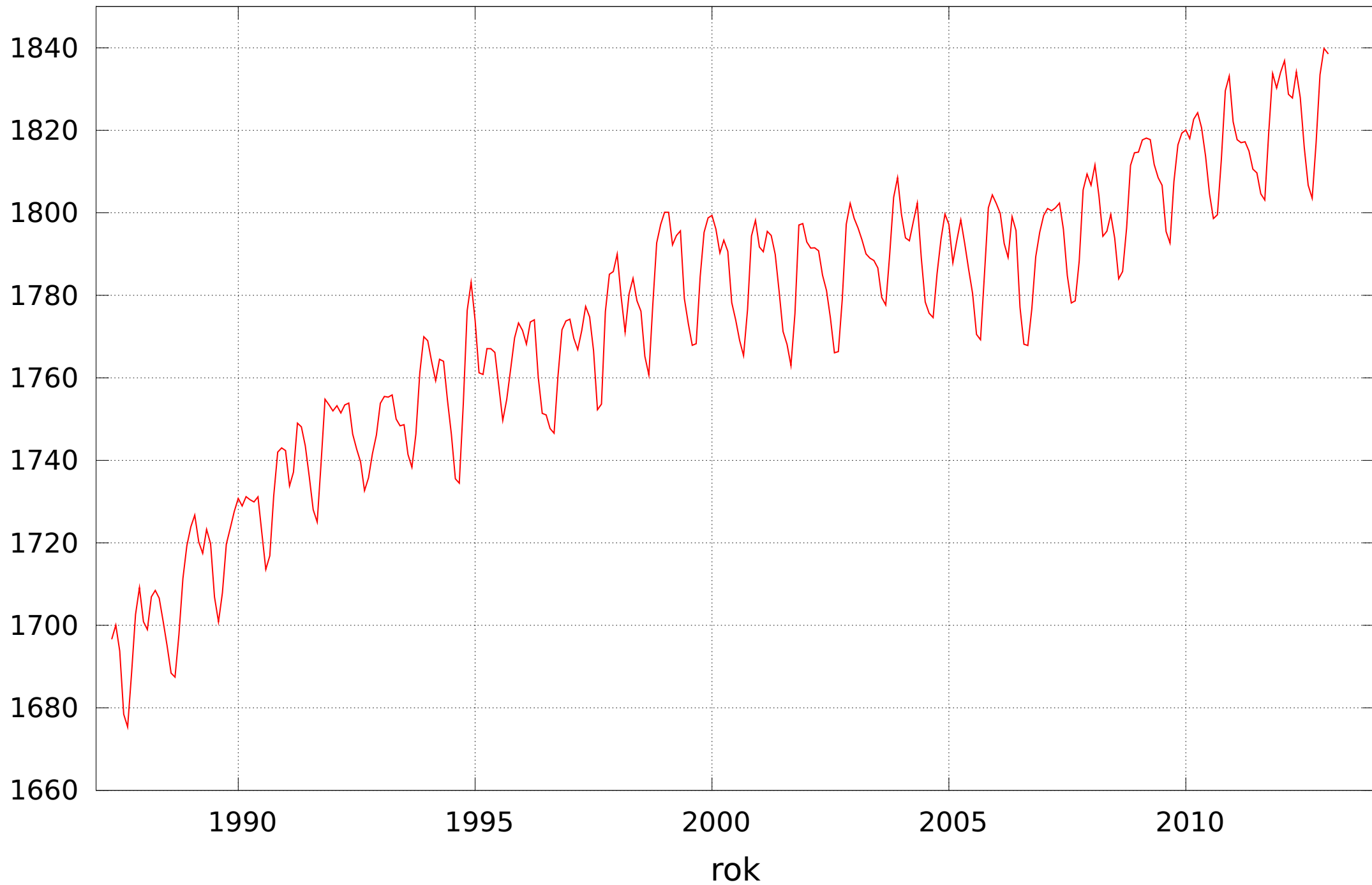
Koncentrace metanu / 1 ppb; měsíční průměry z Mauna Loa
