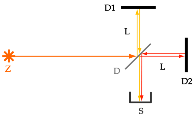
Obr. 4: Schéma Michelsonova pokusu
