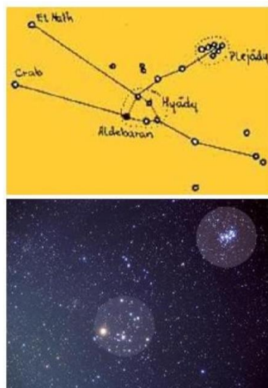
Obr. 130: Hyády – schéma a fotografie souhvězdí Býka
