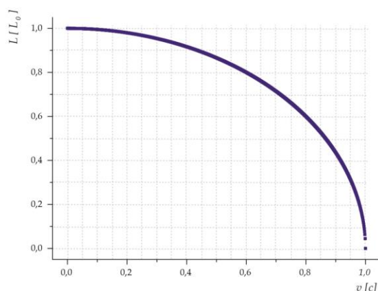
Obr. 40: Kontrakce délek – na vodorovné ose je zanesena rychlost pohybu (ve zlomcích rychlosti světla), na svislé ose kontrahovaná délka (ve zlomcích délky klidové)
