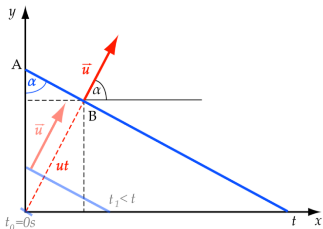
Obr. 19: Relativistická aberace světla – náčrtek pro odvození
