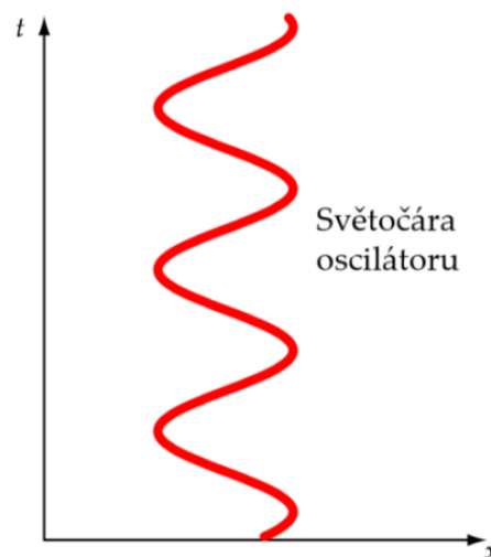
Obr. 31: Světočára oscilátoru kmitajícího podél osy x
