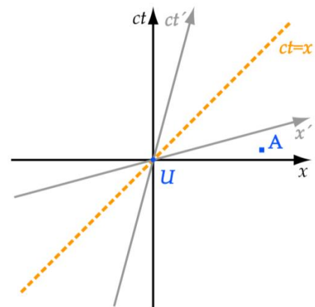
Obr. 33: Lorentzova transformace v prostoročasovém diagramu
