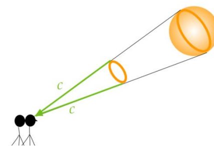
Obr. 16: Pozorovaný obrys koule dvěma pozorovateli
