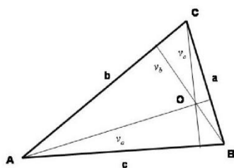
Obr.115: výšky v trojúhelníku se protínají v jediném bodě.
