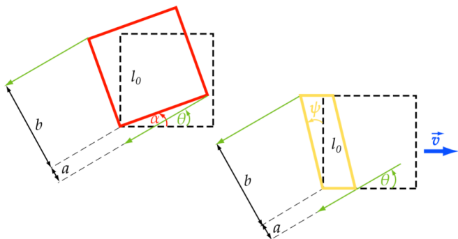
Obr. 14: Čtverec – otočení a skutečný tvar
