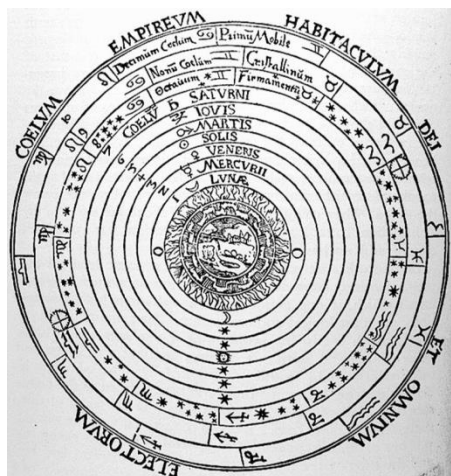
Obr. 48: Představa o sluneční soustavě podle Aristotela
