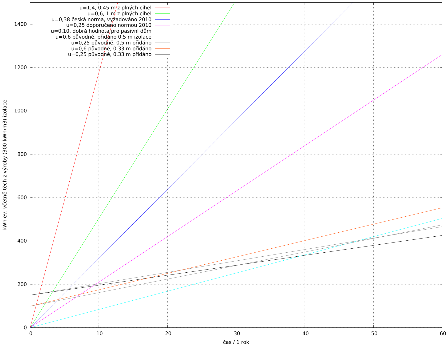
Teplo skrze 1 m2 zdi během topných období (3500 d.K/a), s/bez přidané izolace ( \lambda=0,035 \text{ W}/(\text{m.K}) )
