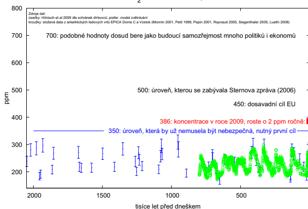
Koncentrace CO 2 během čtvrtohor, dnes a ...zítra?
