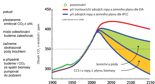
Dosažitelný vývoj koncentrací CO 2
