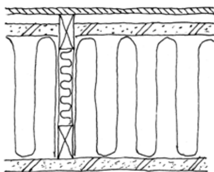
Figur 33. Vægkonstruktioner.
