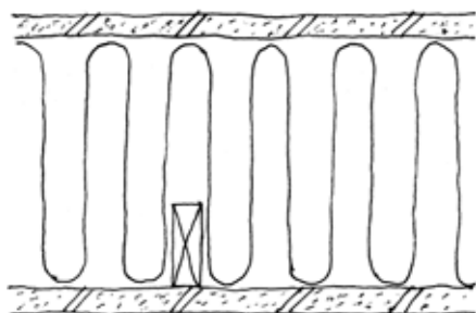
c Ler- eller kalkpuds Halmballer Træstolper mellem halmballer Lerpuds.
