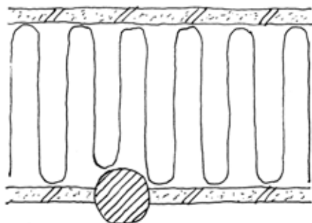
b Ler- eller kalkpuds Halmballer Lerpuds Træstolper, delvis i væg.
