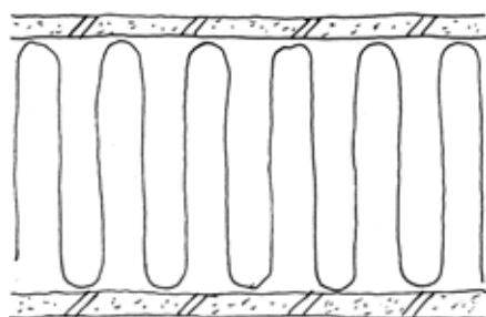
a Ler- eller kalkpuds Halmballer Lerpuds Træstolper, fritstående.
