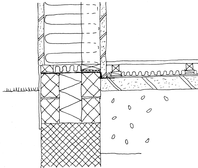
Figur 35. Skjult trækonstruktion på sribefundament ca. 1:20. Der indlægges drænende isolering over fugtspærren i fundamentet. Når fugtspærren i fundamentet forbindes til fugtspærren på gulvet sikres samtidig tæthed mod radon.
