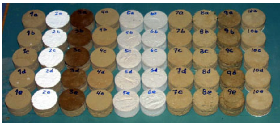
Figur 41. Vanddamppermeabiliteten testes ved kopforsøg på 10 forskellige materialesammensætninger. Numrene svarer til emnenumrene i table 3.
