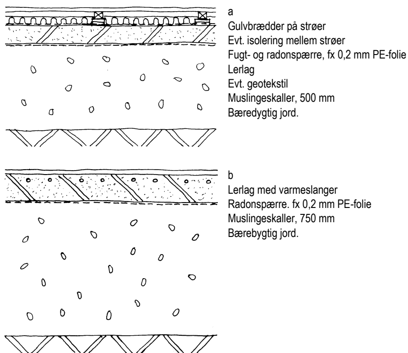
Figur 27. Gulvkonstruktioner isoleret med muslingeskaller.
