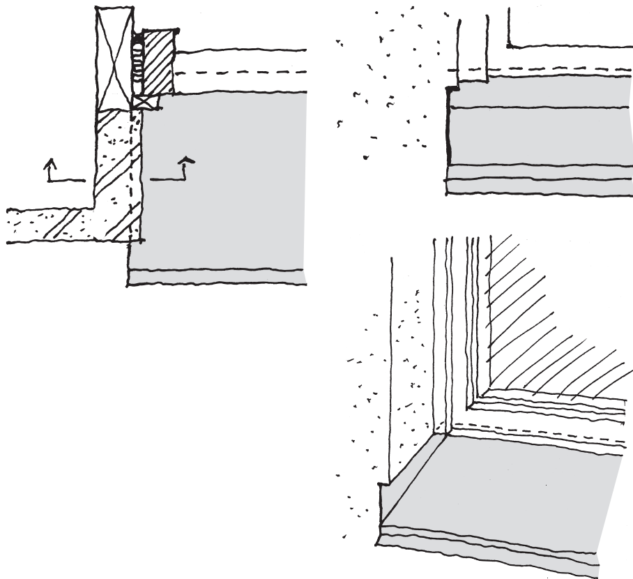
Figur 31. Princip for udformning af sålbænk. Sålbænkens endebund er forsynet med en ombukning for oven, som pudsen kan stå på. Derved undgås det, at pudsen står på sålbænkens bund, hvor den kan opsuge vand.
