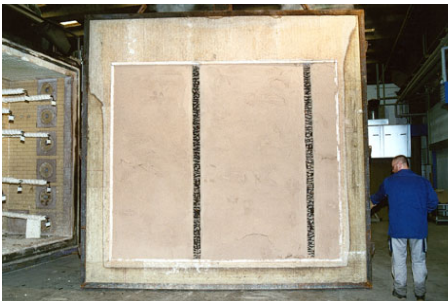
Figur 50. Lerpudset halmvæg anvendt ved bestemmelse af brandmodstandsevne. Det bemærkes specielt, at der ikke er sket indbrænding mellem træstolperne og pudsens overflade.
