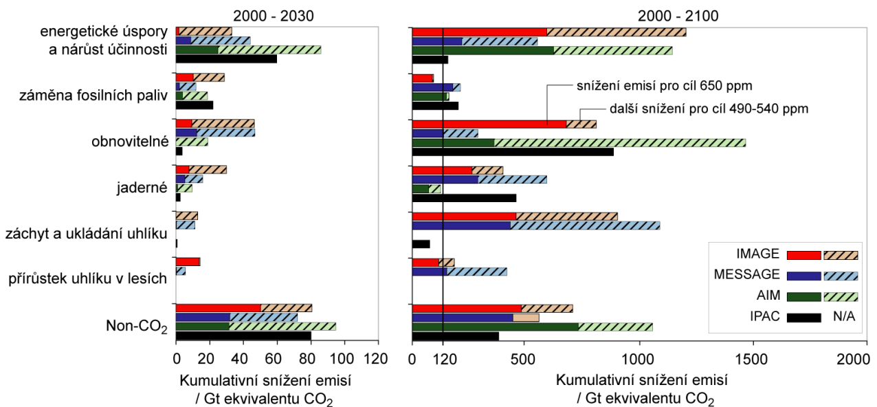
Obrázek SPM 9: Kumulativní snížení emisí u alternativních opatření zmírňování pro období let 2000 – 2030 (levá část) a pro období let 2000 – 2100 (pravá část). Obrázek ukazuje ilustrativní scénáře ze čtyř modelů (AIM, IMAGE, IPAC a MESSAGE) zaměřených na stabilizaci ekv. CO 2 na úrovni 490-540 ppm a na úrovni 650 ppm. Tmavé úsečky znázorňují snížení pro cílovou hodnotu ekv. CO 2 650 ppm a jejich světlé pokračování další žádoucí snížení pro dosažení hodnoty 490-540 ppm. Stojí za zmínku, že některé modely neberou v úvahu zmírňování pomocí zvýšeného pohlcování uhlíku lesními ekosystémy (AIM a IPAC) nebo CCS (AIM), a že podíl nízkouhlikových energetických alternativ na celkových dodávkách energií je také určován zahrnutím těchto možností do referenční úrovně. CCS zahrnuje zachycování a ukládání uhlíku z biomasy. Pohlcování uhlíku lesními ekosystémy zahrnuje pokles emisí z odlesňování [Obrázek 3.23].
