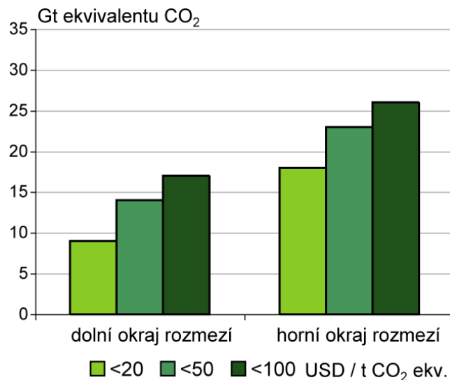
Obrázek SPM.5B: Globální ekonomický potenciál zmírňování v roce 2030 odhadovaný pomocí studií „shora dolů“ (údaje z Tabulky SPM.2)
