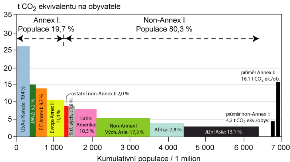
Obrázek SPM.3a: Rozložení regionálních emisí skleníkových plynů na obyvatele v roce 2004 (všechny plyny dle Kjótského protokolu, včetně plynů z využívání půdy) oproti populaci různých seskupení zemí. Procentuální hodnoty uvedené ve sloupcích představují podíl regionů na globálních emisích skleníkových plynů [Obrázek 1.4a].
