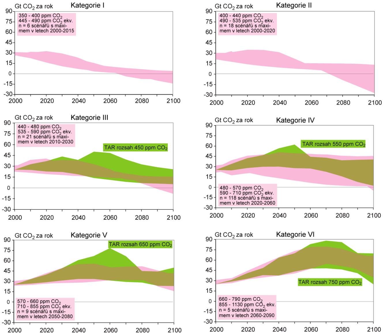
Obrázek SPM.7: Vývoj emisí u mitigačních 1 scénářů pro alternativní kategorie úrovní stabilizace (kategorie I – VI definované v rámečku u každého panelu). Tyto vývojové trendy jsou znázorněny pouze pro emise CO 2 . Růžové plochy znázorňují emise CO 2 pro emisní scénáře publikované po vydání Třetí hodnotící zprávy (TAR). Zelené plochy představují rozsah více než 80 stabilizačních scénářů Třetí hodnotící zprávy (TAR). Emise výchozího roku se u jednotlivých modelů mohou v důsledku rozdílů v pokrytí sektorů a průmyslu lišit. Pro dosažení nižších stabilizačních úrovní uplatňují některé scénáře odstraňování CO 2 z atmosféry (negativní emise) pomocí takových technologií jako např. výroby energie z biomasy s využitím zachycování a ukládání uhlíku [Obrázek 3.17].
