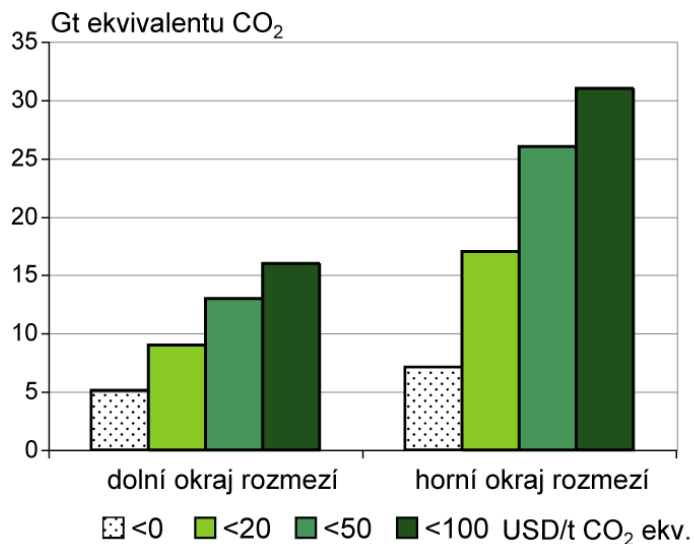
Obrázek SPM.5A: Globální ekonomický potenciál zmírňování v roce 2030 odhadovaný pomocí studií „zdola nahoru“ (údaje z Tabulky SPM.1).
