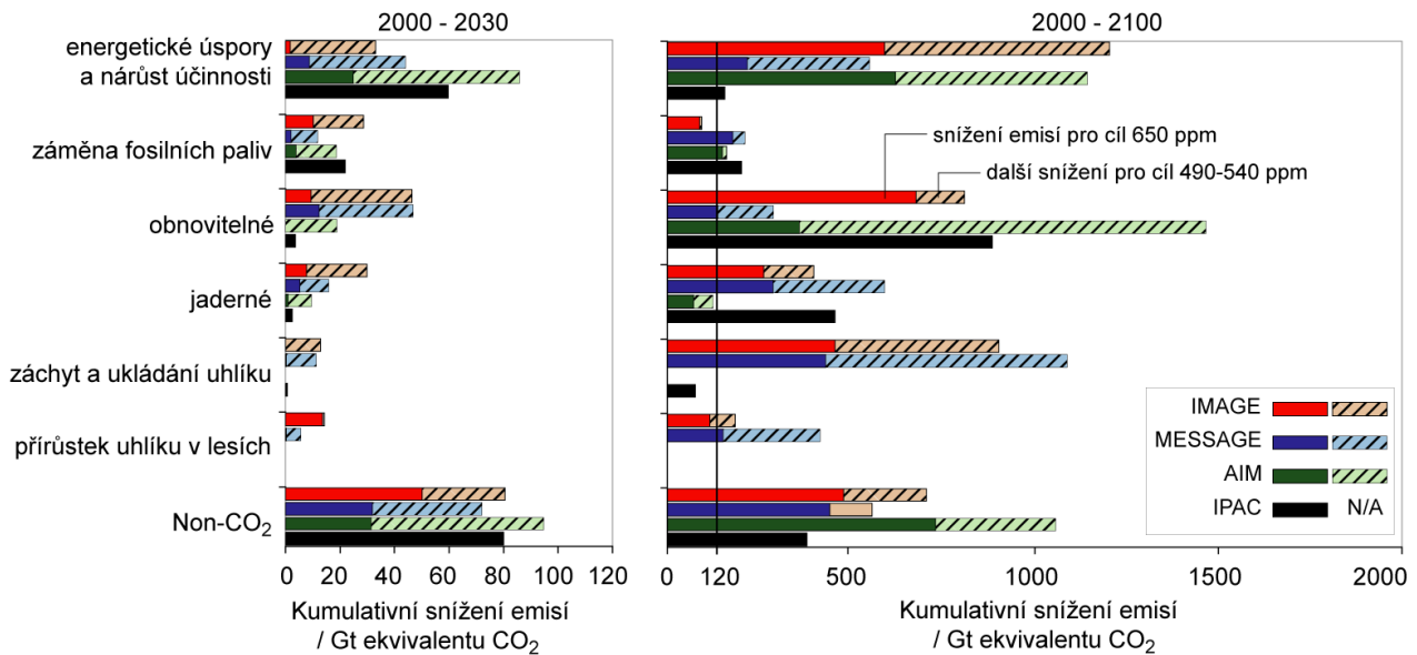
Obrázek SPM.9: Kumulativní snížení emisí při různých způsobech zmírňování pro období let 2000 – 2030 (levá část) a pro období let 2000 – 2100 (pravá část). Obrázek ukazuje ilustrativní scénáře ze čtyř modelů (AIM, IMAGE, IPAC a MESSAGE) zaměřených na stabilizaci ekvivalentu CO 2 na úrovni 490 ppm až 540 ppm a na úrovni 650 ppm a jejich světlé pokračování další žádoucí snížení pro dosažení hodnoty 490–540 ppm. Stojí za zmínku, že některé modely neberou v úvahu zmírňování pomocí zvýšeného pohlcování uhlíku lesními ekosystémy (AIM a IPAC) nebo CCS (AIM), a že podíl nízkouhlíkových energetických alternativ na celkových dodávkách energií je také určován zahrnutím těchto možností do referenční úrovně. CCS zahrnuje zachycování a ukládání CO 2 z biomasy. Pohlcování uhlíku lesními ekosystémy zahrnuje pokles emisí z odlesňování [Obrázek 3.23].
