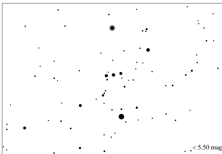
Mapky pro Globe at Night. 22. března ve 20 h (začátek astronomické noci) je Orionův pás 30^\circ vysoko, Betelgeuze 40^\circ . Spočteno pro velmi průzračný vzduch (extinkce v zenitu 0,20 mag). J. Hollan, Hvězdárna a planetárium Mikuláše Koperníka v Brně, http://globe.hvezdarna.cz
