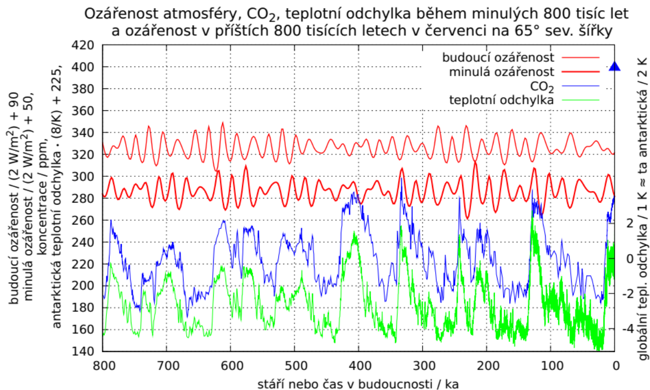
Obrázek 3.1: Červené křivky udávají proměny intenzity ozáření (aneb ozáření) vodorovné plochy ovzduší poblíž polárního kruhu v červenci. Tlustě jsou vyznačeny hodnoty minulé, tenké budoucí. Koncentrace oxidu uhličitého i teplotní anomálie jsou zjištěné z ledových vrtných jader v Antarktidě; antarktické teplotní odchylky jsou zhruba dvojnásobkem anomálií globálních. Koncentrace CO 2 v r. 2015, 400 ppm, je vyznačena modrým trojúhelníkem. (K popiskům: „ka“ je tisíc let, „a“ je značka pro rok z latinského annus ; změní-li se antarktická teplota o dva kelviny, globální se změní jen o jeden kelvin)
