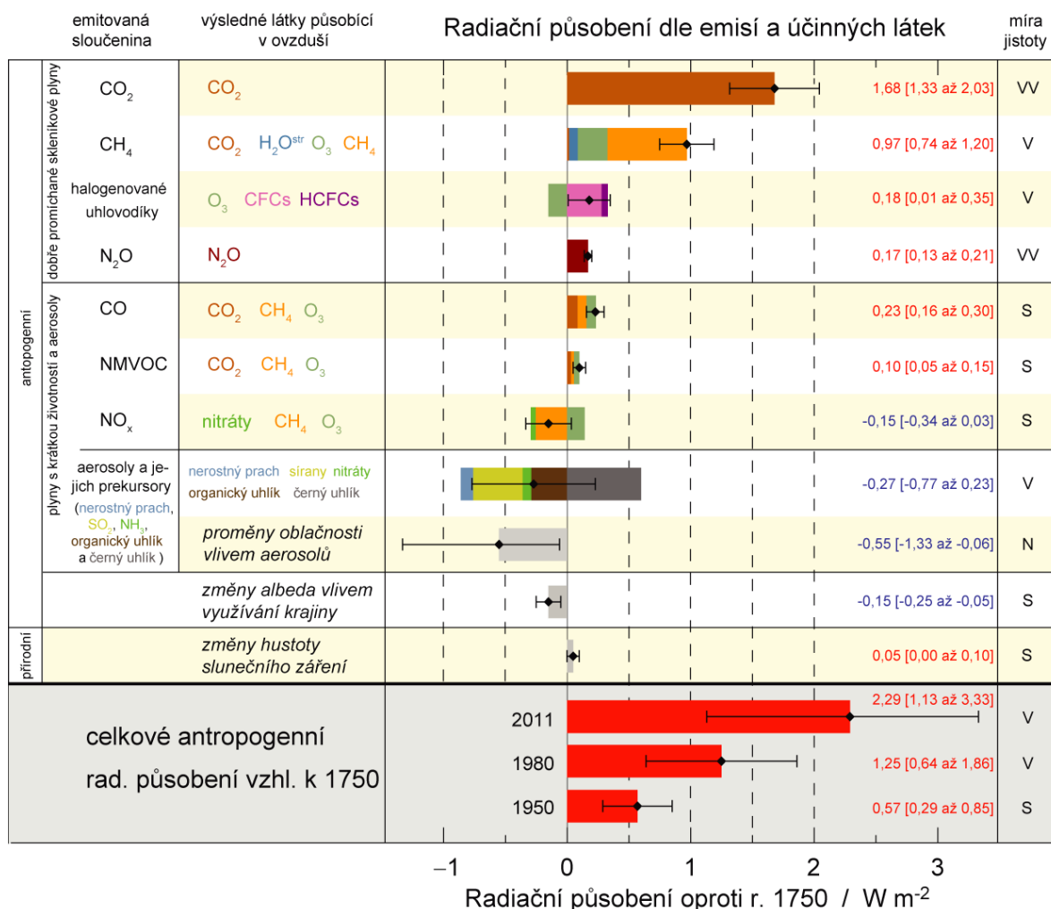
Obrázek 2.9: Oteplovací vliv různých látek přidávaných do ovzduší. Česká verze obrázku SPM 5 prvního dílu (Fyzikální základy) Páté hodnotící zprávy IPCC; tento a další obrázky Shrnutí pro politické představitele: http://amper.ped.muni.cz/gw/ipcc_cz/ar5/Fyzikalni_zaklady/figures_cz/ .
