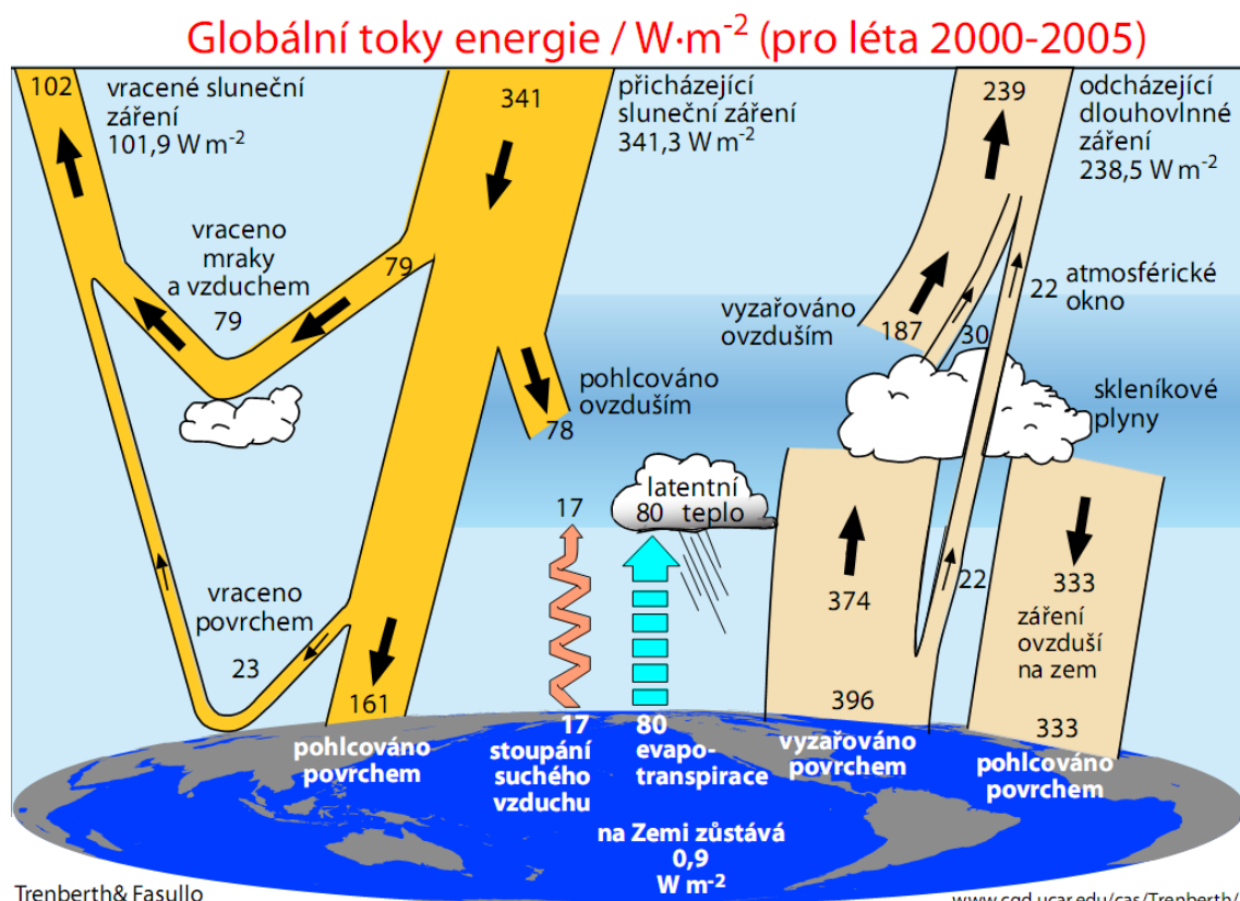
Obrázek 2.10: Toky energie ovzduším Země, bráno globálně
