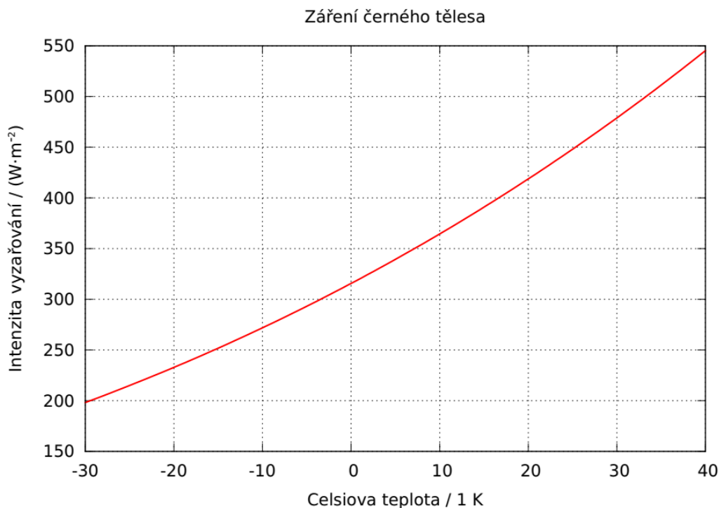
Obrázek 2.1: Intenzita vyzařování (angl. radiant exitance) „černého tělesa“ v závislosti na jeho Celsiově teplotě. Dle Stefanova-Boltzmannova zákona činí 5,67 \cdot 10^{-8} \text{ W}\cdot\text{m}^{-2} \text{ K}^{-4} T^4 , kde T je absolutní teplota, tedy Celsiova teplota + 273,15 K. ( zdrojový skript )
