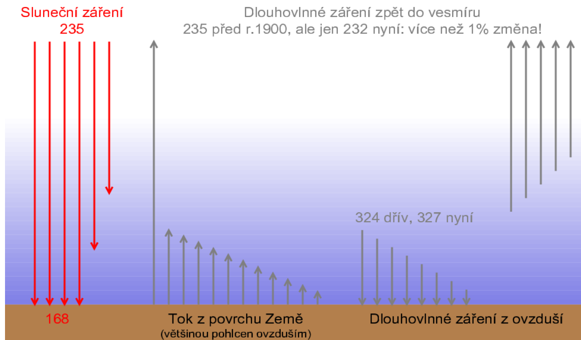
Obrázek 2.2: Schéma skleníkového jevu pro rok 2000 pro hypotetickou situaci, že by Země byla stejně teplá jako před průmyslovou revolucí. Začátky a konce šipek, nejsou-li „na povrchu“ nebo „ve vesmíru“, naznačují, odkud z ovzduší záření vychází a kde je jím pohlcováno. Počet šipek symbolizuje úhrn tepelného toku, každá šipka představuje 40 \text{ W/m}^2 .
