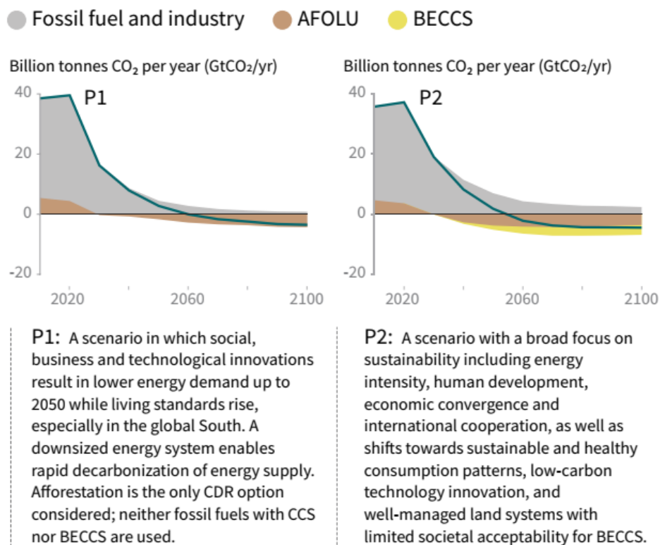
Obrázek 6.2: Výřez z obrázku SPM.3b zprávy Global Warming of 1.5 °C ukazující dvě alternativy, jak ohromně rychle by musely klesat emise oxidu uhličitého, aby nárůst teploty úroveň 1,5 K nepřekročil nebo ji překročil jen na krátkou dobu. Na svislé ose jsou emise CO 2 v gigatunách za rok.
